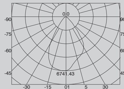
Valores de Intensidad Luminosa en cd/klm
